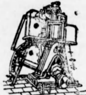
Szivógázmotortelep. — A jelenkor legelőcsöb üzema „Benzin” nyersolajmotor.
